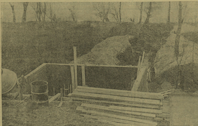
Obras de la casa de máquinas para la toma de agua del Regadío de Baños de Ebro
