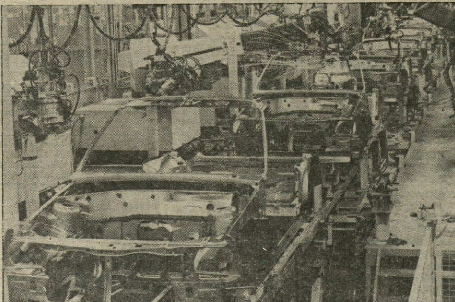
Todo está automatizado. Los robots se encargarán de hacer los movimientos precisos para establecer los puntos exactos de soldadura.
